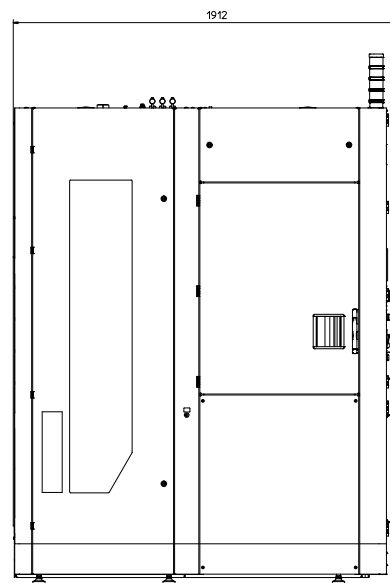
Seitenansicht
