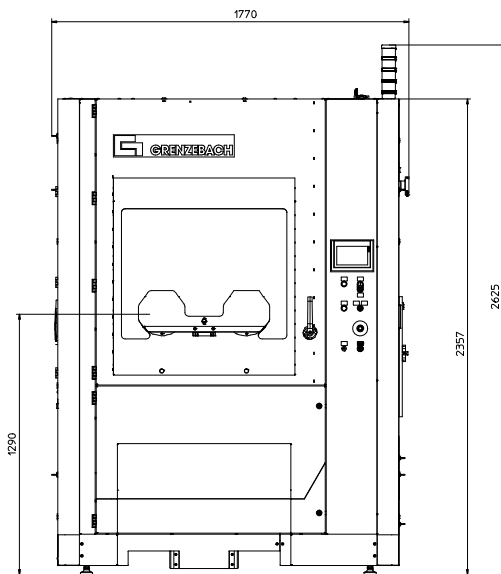
Vorderansicht
